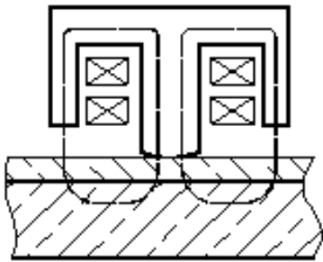
磁性法基本工作原理
