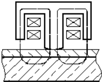
磁性法基本工作原理
